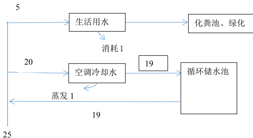
图 1 全厂水平衡图 (单位: m 3 /d)
