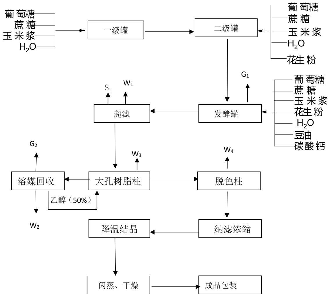
图 4.3-1 7-ACA 合成生产工艺流程及排污环节图
