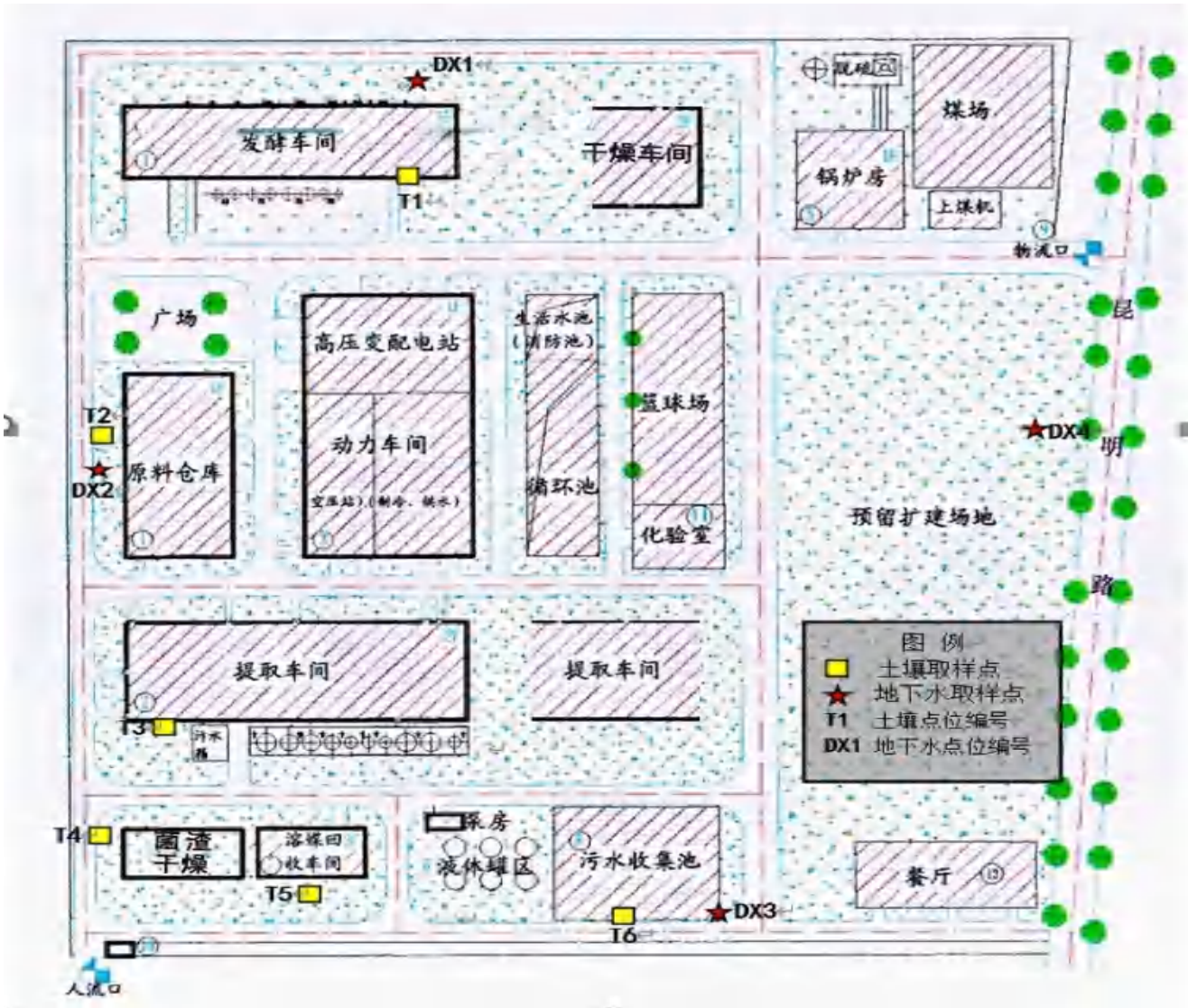
图 6.1-1 土壤和地下水监测点位设置平面
